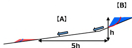
【腹付け盛土】
